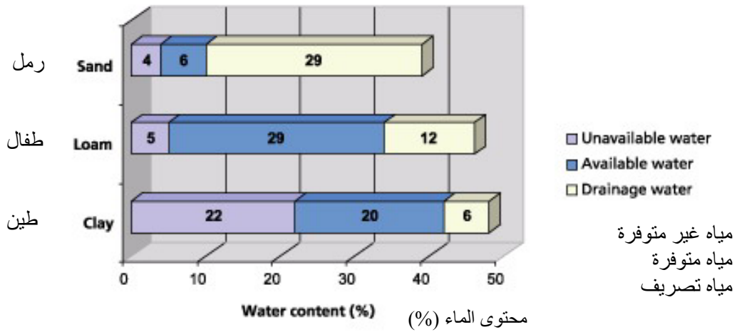
الشكل 3.4 : فراغ التربة في ثلاث ترب مختلفة وقدرتها على الاحتفاظ بالماء.
