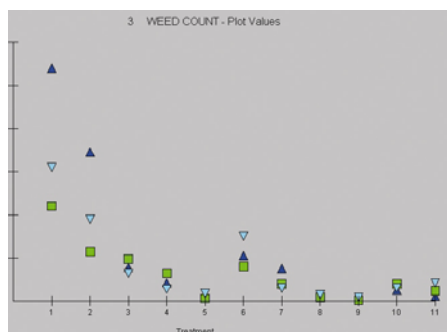
تحويل لوغاريتمي
