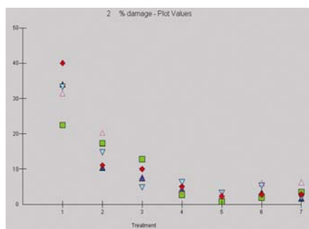
تحويل أركسايين
