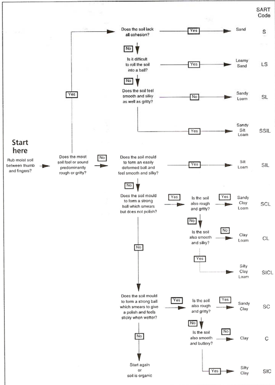
شكل 3.17. مفتاح تصنيفي لتركيب التربة.
