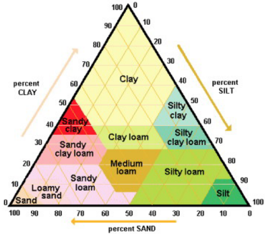
شكل 3.16. رسم بياني لتحديد قوام التربة تبعاً لحجم جزيئات التربة المختلفة. (clay = طين "وحد"، loam = طفال، sand = رمل، silt = غرين "طمي").
