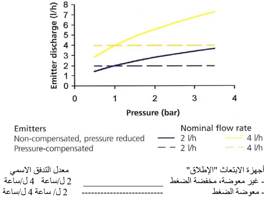
الشكل 3.13: أجهزة ابتعاث "إطلاق" الري بالتنقيط: الضغط مقابل التصريف أو الإطلاق.
